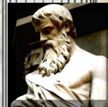
Евклид
